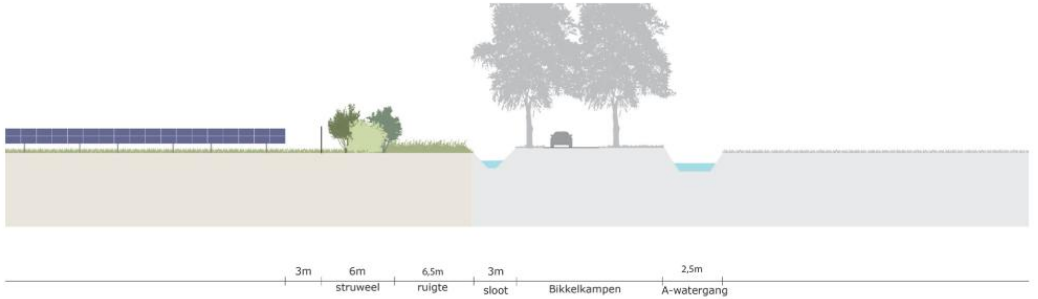
Afbeelding 26 - Dwarsprofiel E-E
