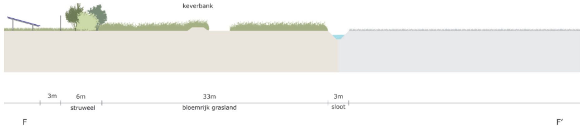
Afbeelding 28 - Dwarsprofiel F-F'
