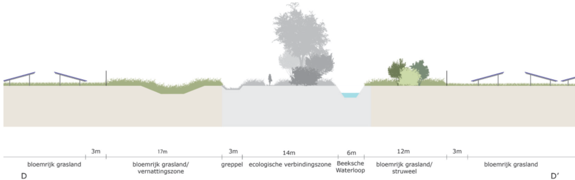
Afbeelding 25 - Dwarsprofiel D-D'
