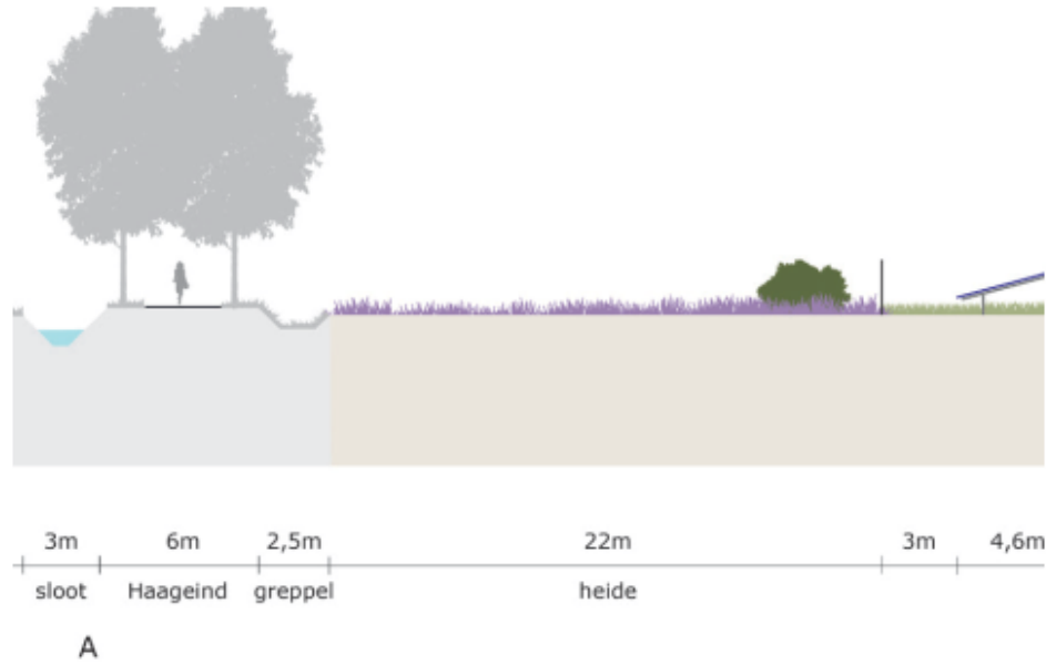
Afbeelding 23 - Dwarsprofiel A-A'
