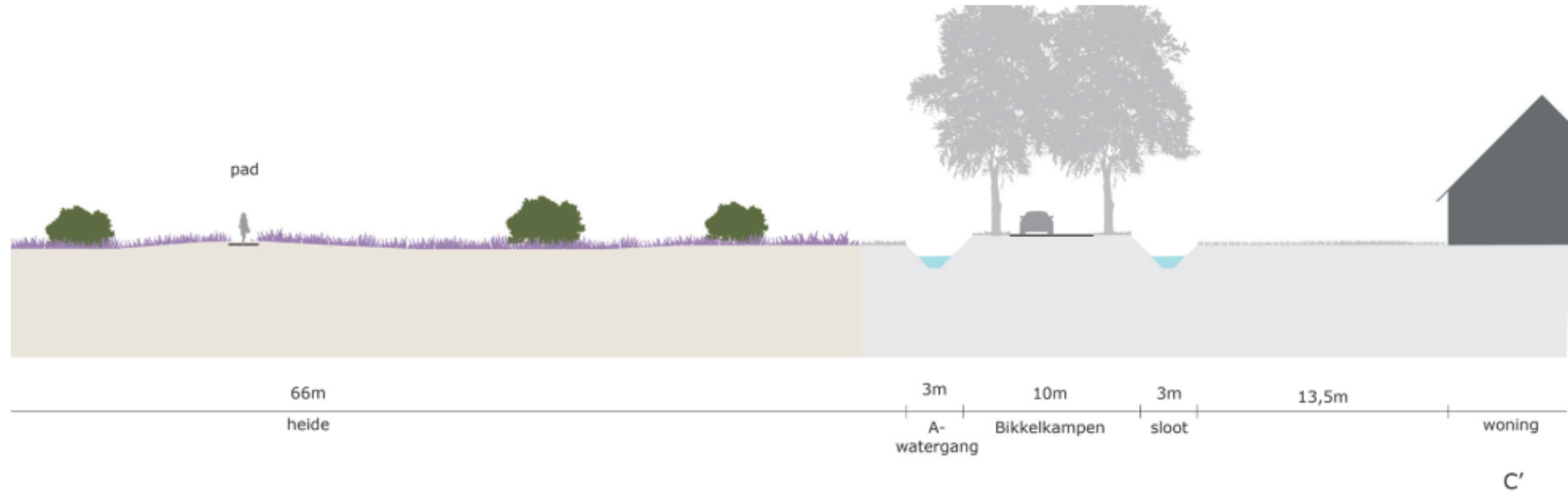
Afbeelding 27 - Dwarsprofiel C-C'
