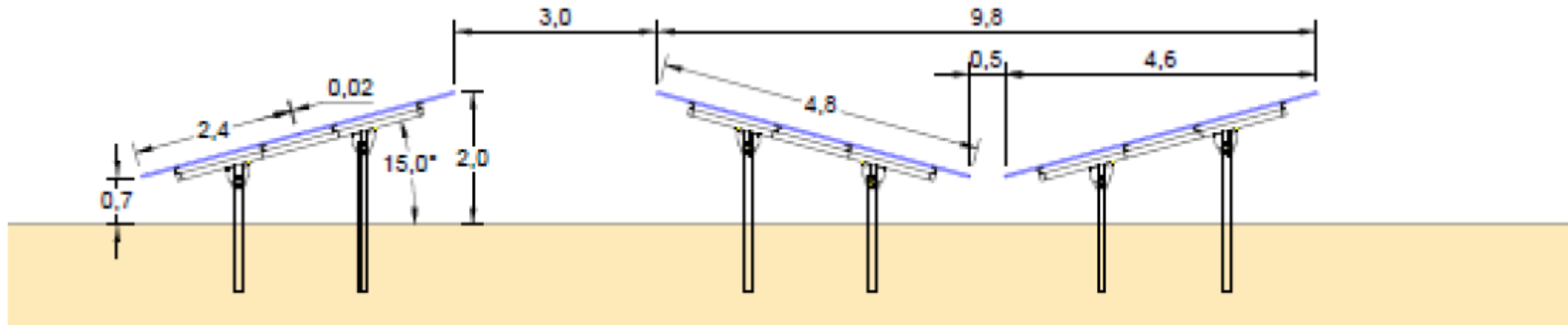
FIGUUR 7: TECHNISCHE TEKENING VAN DE ZOGEHETEN 'VLINDEROPSTELLING' VAN ZONNEPARK BIKKELKAMPEN. BRON: TPSOLAR
