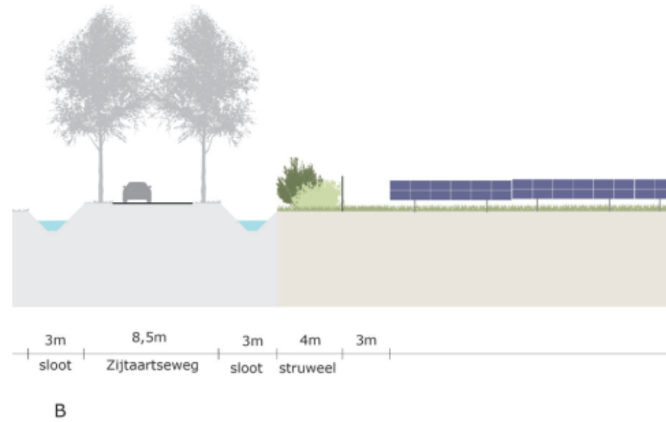
Afbeelding 24 - Dwarsprofiel B-B'
